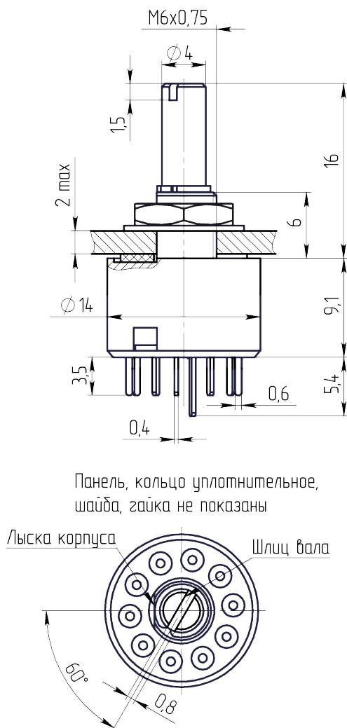
Габаритные и установочные размеры
