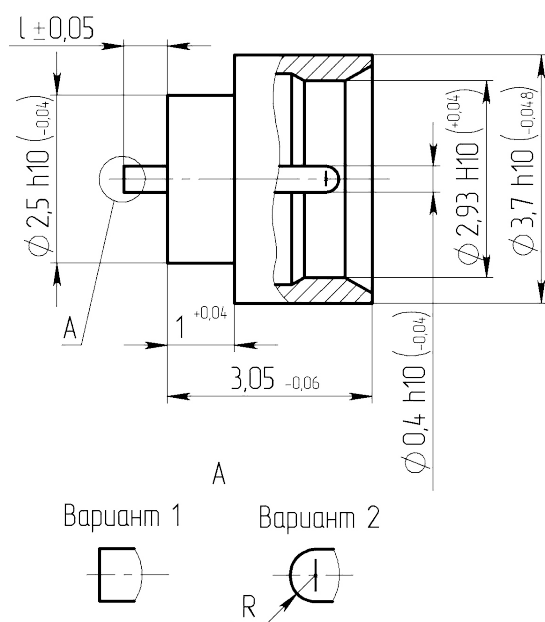
Габаритные и установочные размеры
