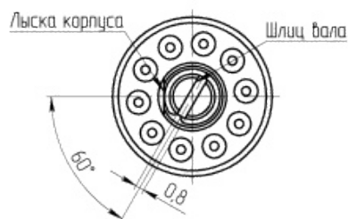
Панель, шайба, гайка не показаны
