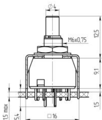
Габаритные и установочные размеры
