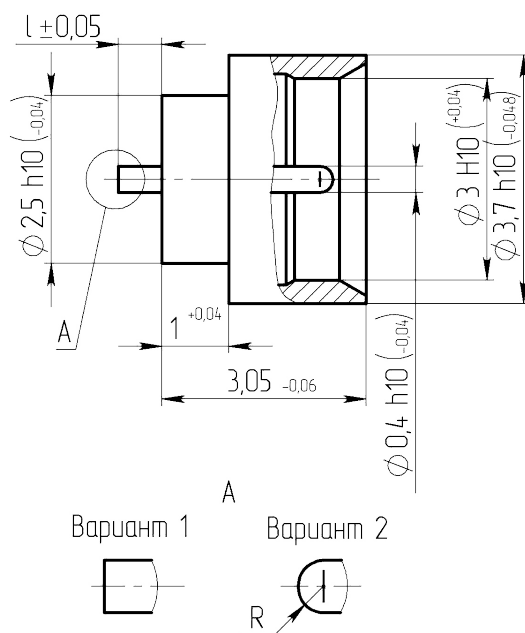
Габаритные и установочные размеры
