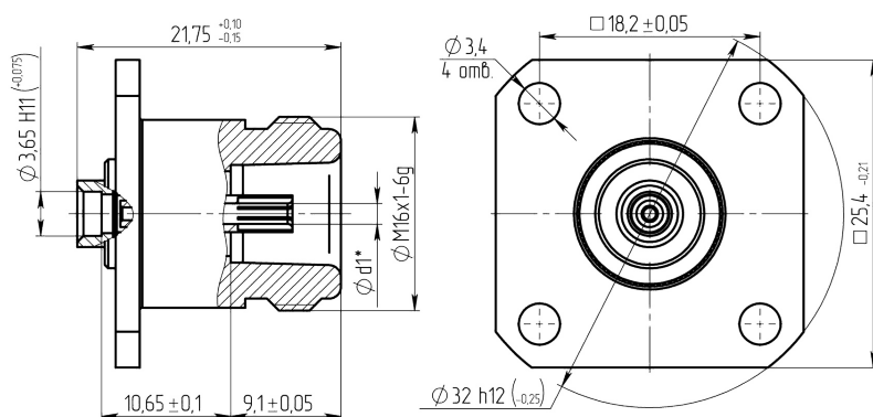
Габаритные и установочные размеры
