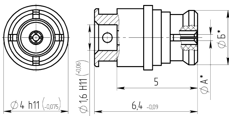
Габаритные и установочные размеры
