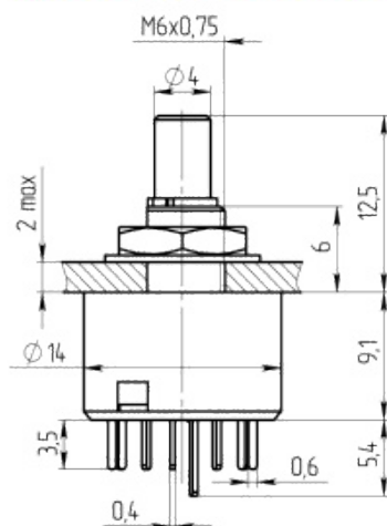
Габаритные и установочные размеры
