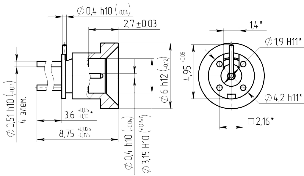
Габаритные и установочные размеры
