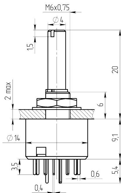
Габаритные и установочные размеры
