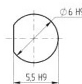
Разметка для крепления на панель
