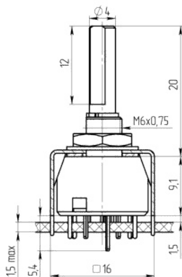
Габаритные и установочные размеры
