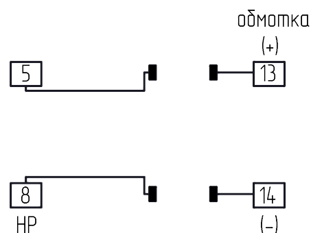
Схема соединения
