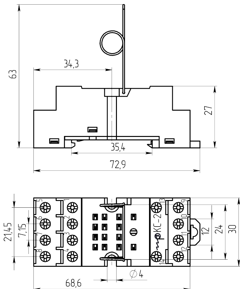
Габаритные и установочные размеры
