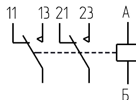
Электрическая принципиальная схема
