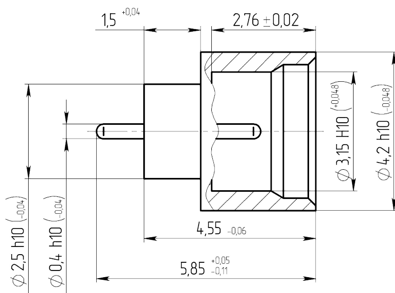
Габаритные и установочные размеры
