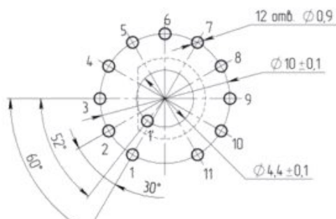
Разметка для крепления на плату (вид со стороны вала)
