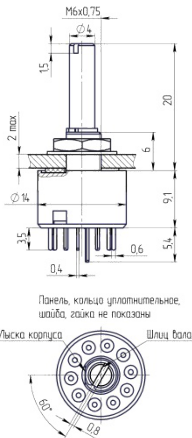
Габаритные и установочные размеры
