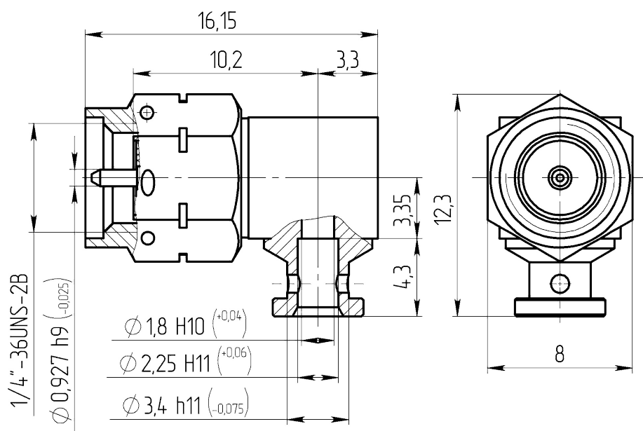
Габаритные и установочные размеры
