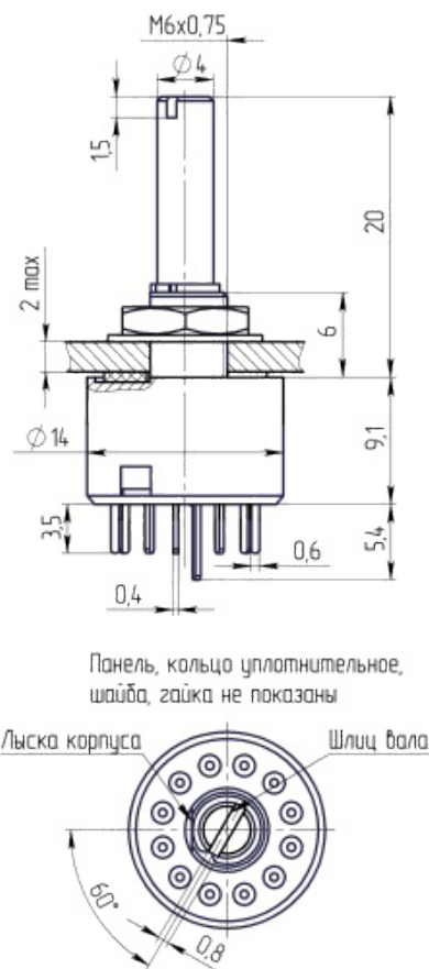
Габаритные и установочные размеры
