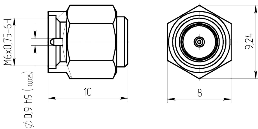
Габаритные и установочные размеры
