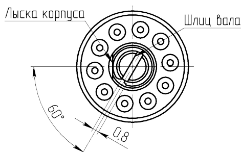
Панель, шайба, гайка не показаны
