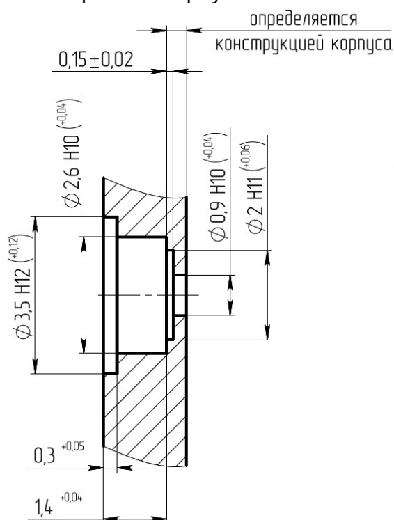
Отверстие в корпусе
