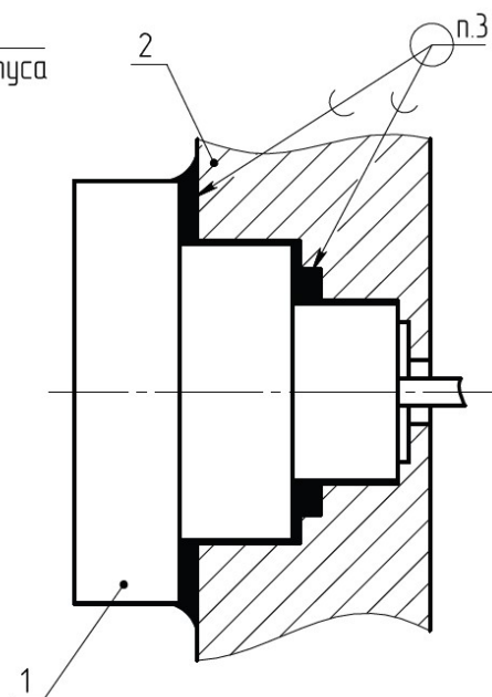
Установка в корпус
