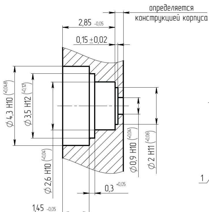
Отверстие в корпусе
