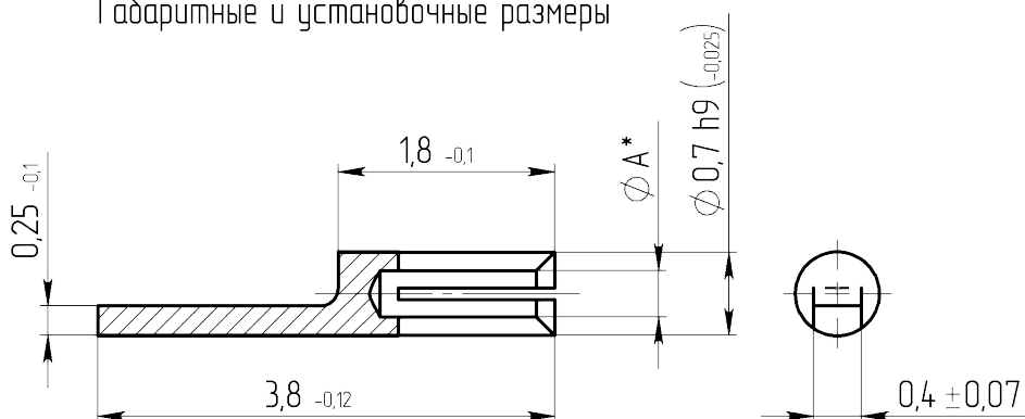
Габаритные и установочные размеры
