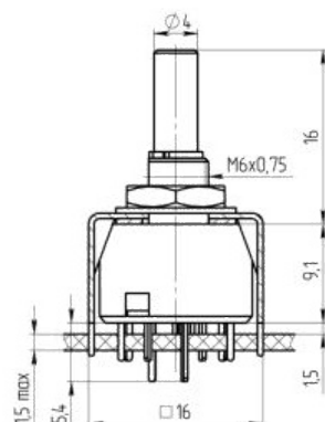
Габаритные и установочные размеры
