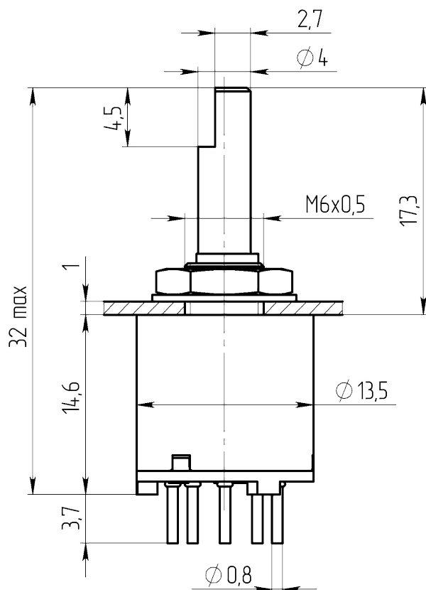
Габаритные и установочные размеры
