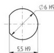
Разметка для крепления на панель
