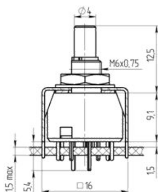
Габаритные и установочные размеры
