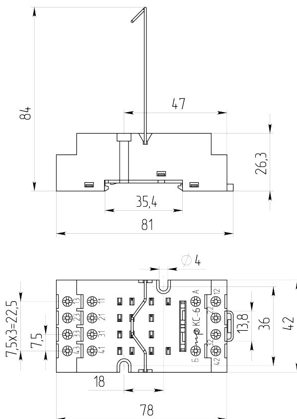
Габаритные и установочные размеры
