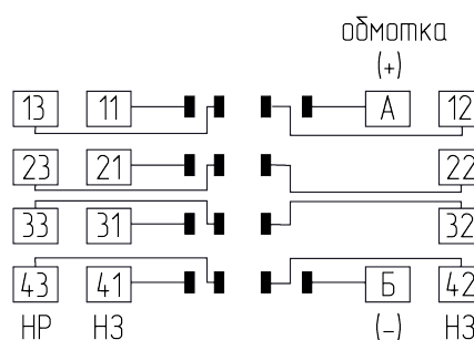
Схема соединения
