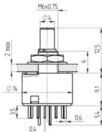
Габаритные и установочные размеры
