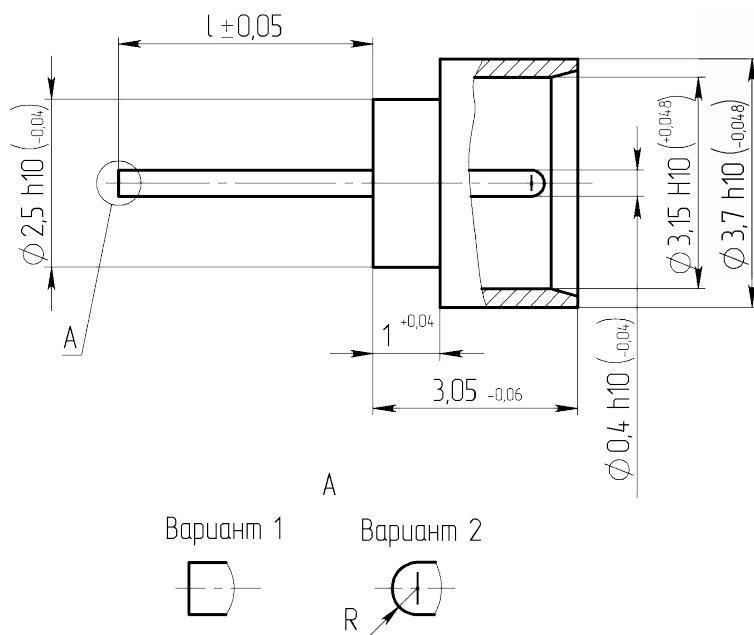
Габаритные и установочные размеры
