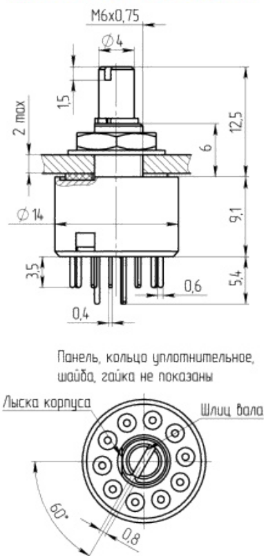
Габаритные и установочные размеры
