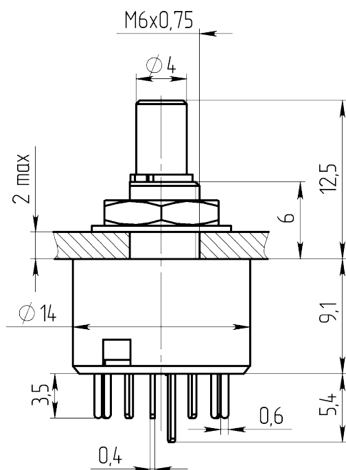
Габаритные и установочные размеры
