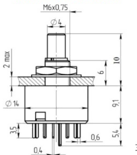
Габаритные и установочные размеры
