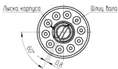
Панель, шайба, гайка не показаны
