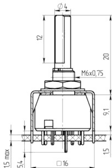
Габаритные и установочные размеры
