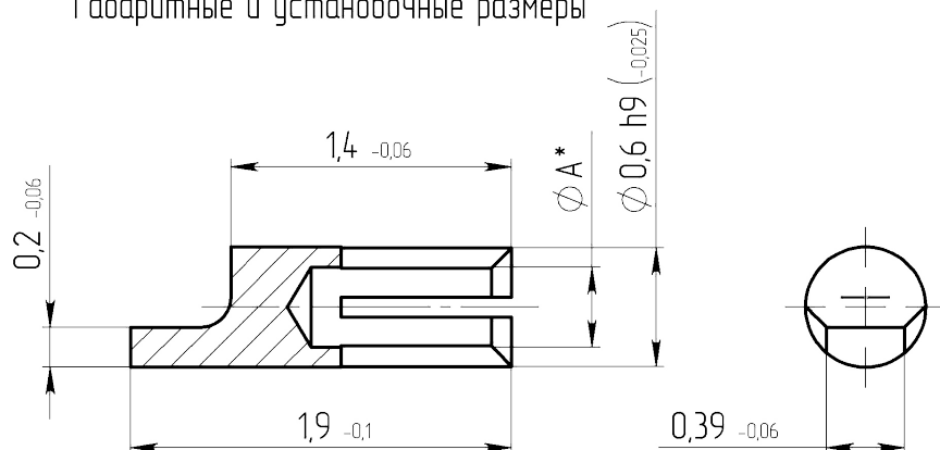
Габаритные и установочные размеры
