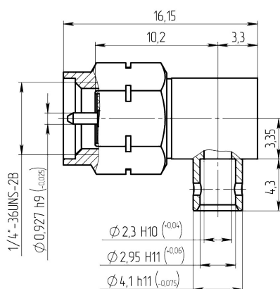
Габаритные и установочные размеры
