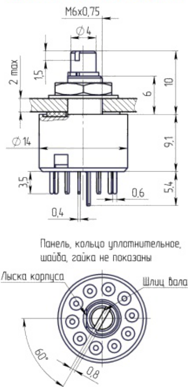
Габаритные и установочные размеры
