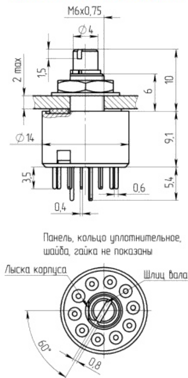
Габаритные и установочные размеры
