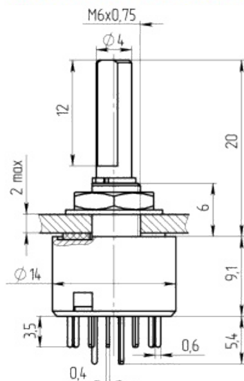
Панель, кольца уплотнительное, шайба, гайка не показаны
