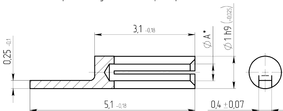
Габаритные и установочные размеры
