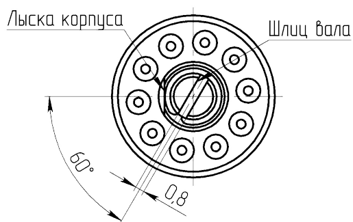
Панель, шайба, гайка не показаны
