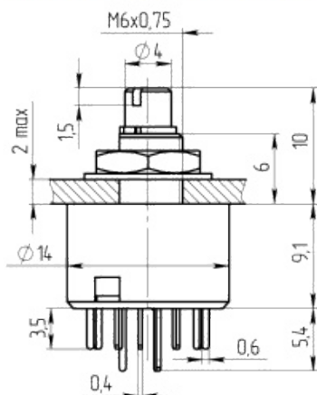
Панель, шайба, гайка не показаны
