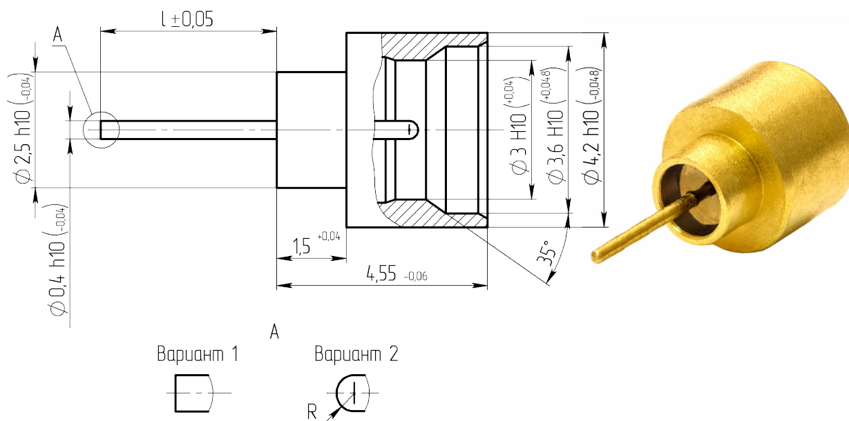
Габаритные и установочные размеры
