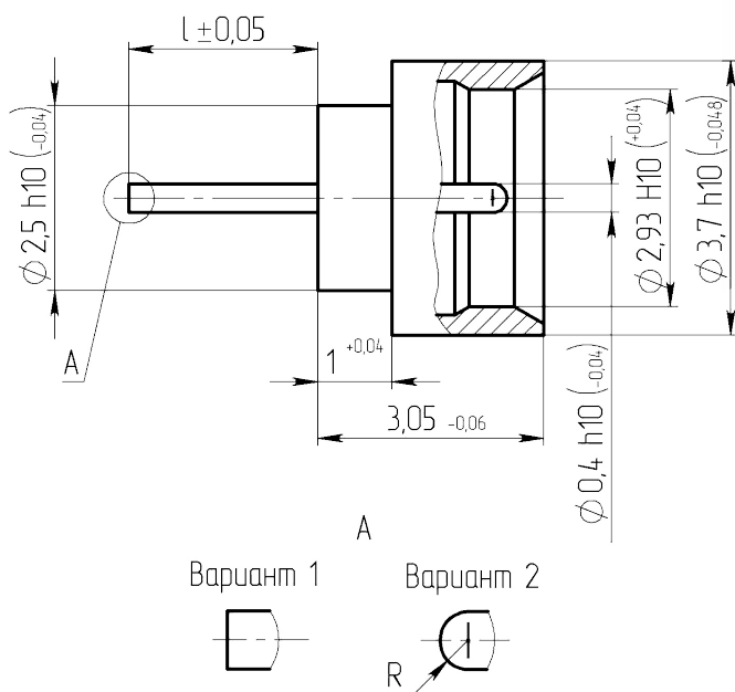
Габаритные и установочные размеры
