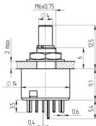
Габаритные и установочные размеры
