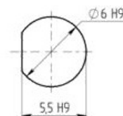
Разметка для крепления на панель
