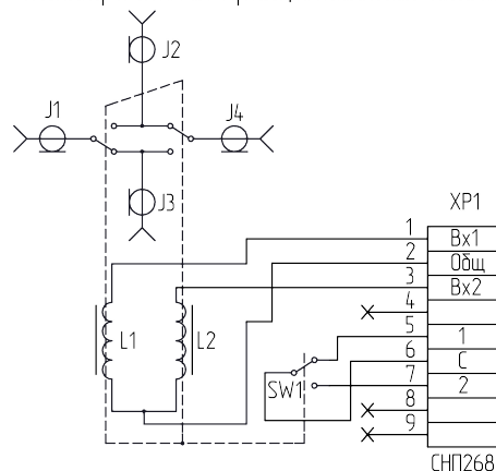
Электрическая принципиальная схема
