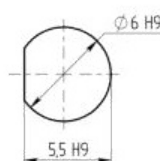
Разметка для крепления на панель
