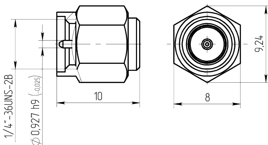
Габаритные и установочные размеры
